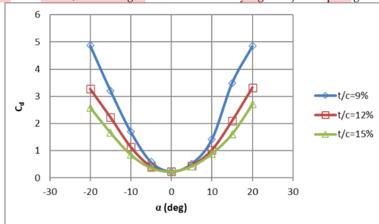
Gambar 5. Grafik hasil komputasi hubungan nilai koefisien drag ( C_d ) model uji terhadap sudut serang ( \alpha ) pada kecepatan free stream 40 m/s untuk setiap tingkat t/c
