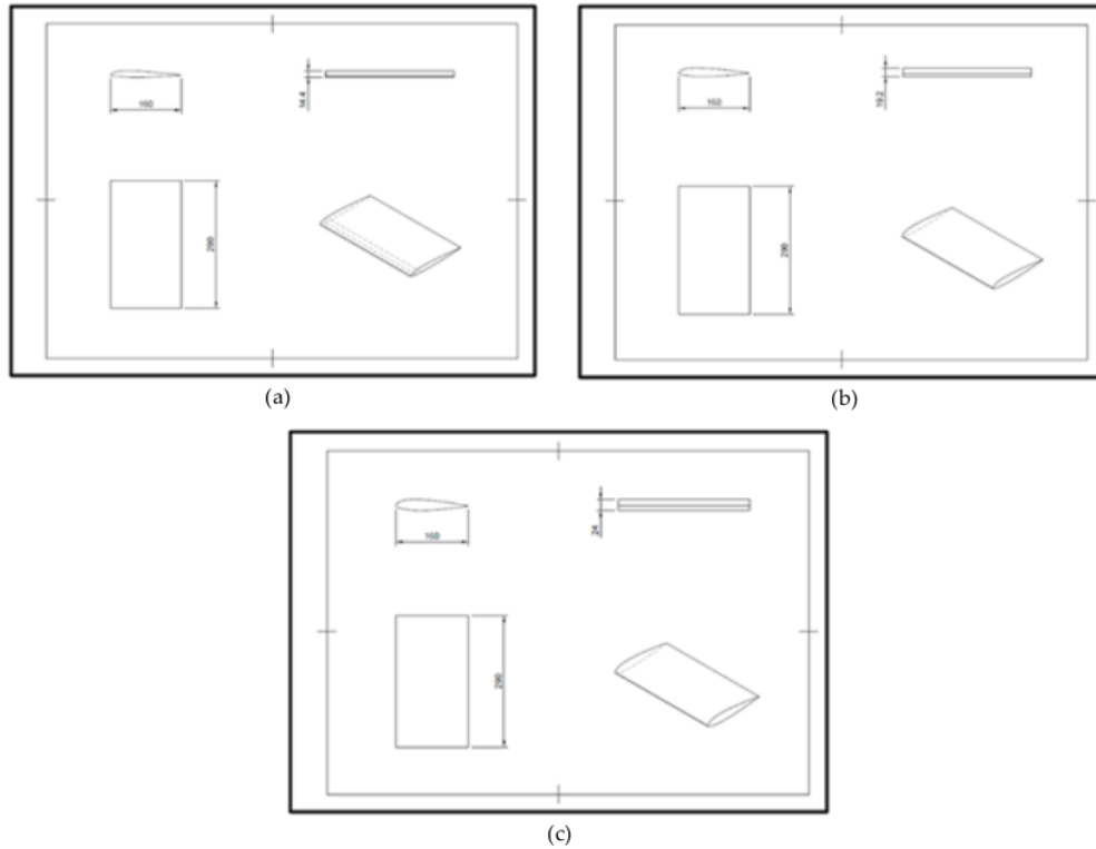
GAMBAR 1. Model uji airfoil dengan (a) model rasio t/c = 9\% , (b) model rasio t/c = 12\% dan (c) model rasio t/c = 15\%
