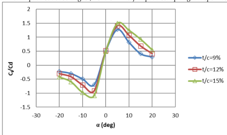
Gambar 7. Grafik hasil komputasi hubungan perbandingan nilai koefisien lift ( C_l ) dengan koefisien drag ( C_d ) atau C_l/C_d model uji terhadap sudut serang ( \alpha ) pada kecepatan free stream 40 m/s untuk setiap tingkat t/c
