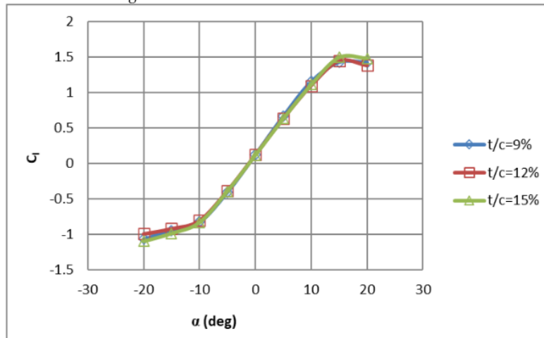
Gambar 4. Grafik hasil komputasi hubungan nilai koefisien lift ( C_l ) model uji terhadap sudut serang ( \alpha ) pada kecepatan free stream 40 m/s untuk setiap tingkat t/c
