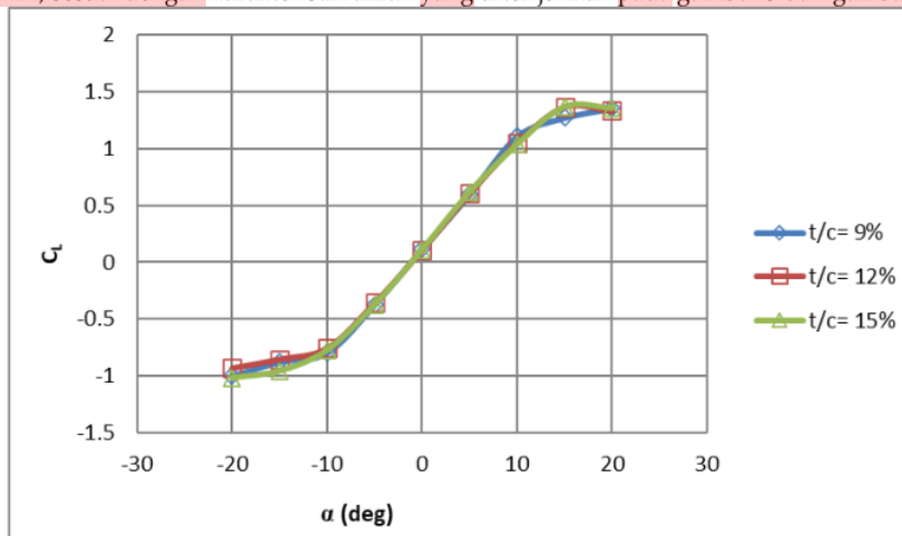
Gambar 6. Grafik hasil eksperimen hubungan nilai koefisien lift ( C_l ) model uji terhadap sudut serang ( \alpha ) pada kecepatan freestream 40 m/s untuk setiap tingkat t/c
