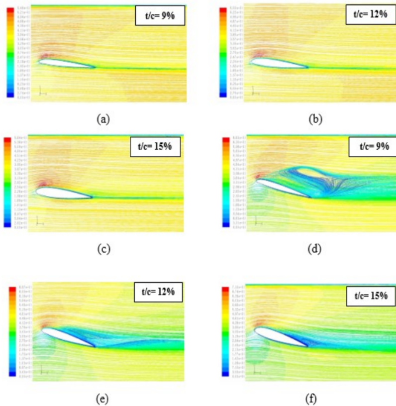
Gambar 3. Pathline kecepatan pada model uji dengan kecepatan free stream 40 m/s, pada sudut serang 5° dengan variasi rasio (a) t/c 9%, (b) t/c 12%, dan (c) t/c 15%, sedangkan pada sudut serang 15° dengan variasi rasio (d) t/c 9%, (e) t/c 12%, dan (f) t/c 15%
